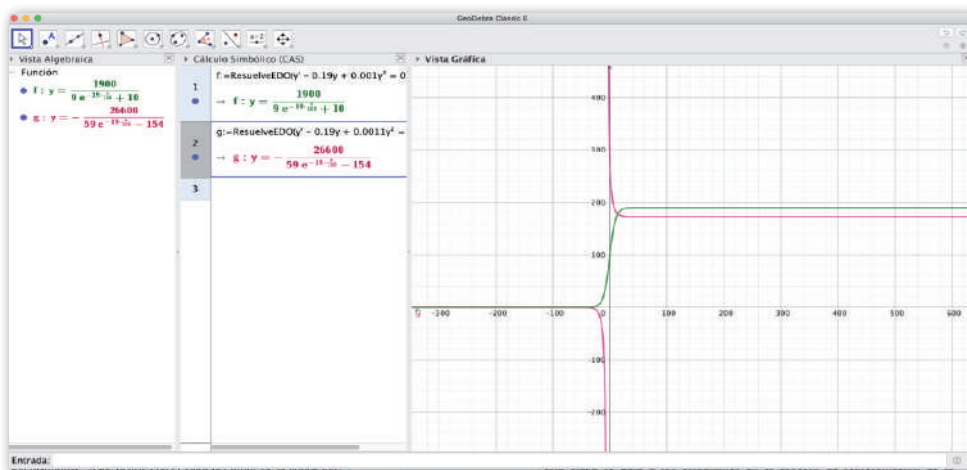
Figura 14. Solución de dos problemas de valores iniciales con diferentes comportamientos
